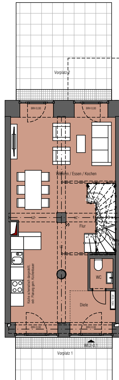
Erdgeschoss
