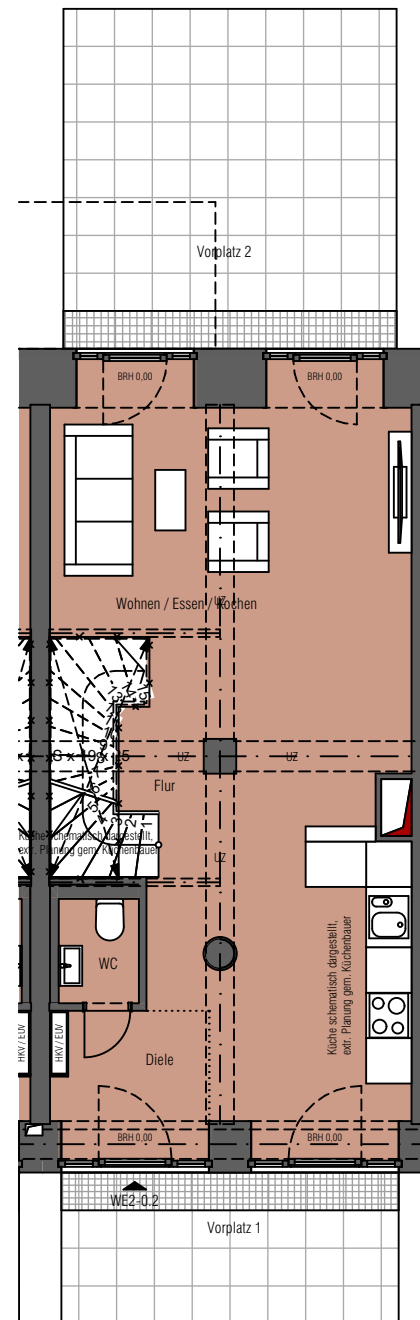
Erdgeschoss
