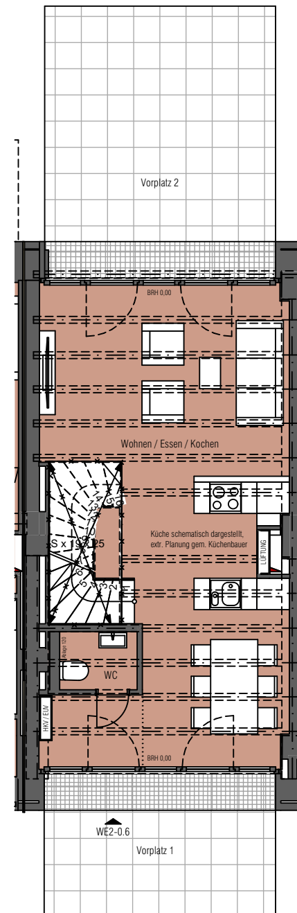
Erdgeschoss
