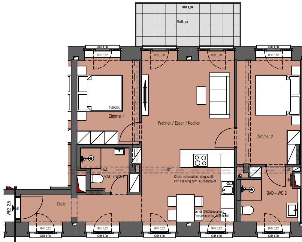
2.Obergeschoss
