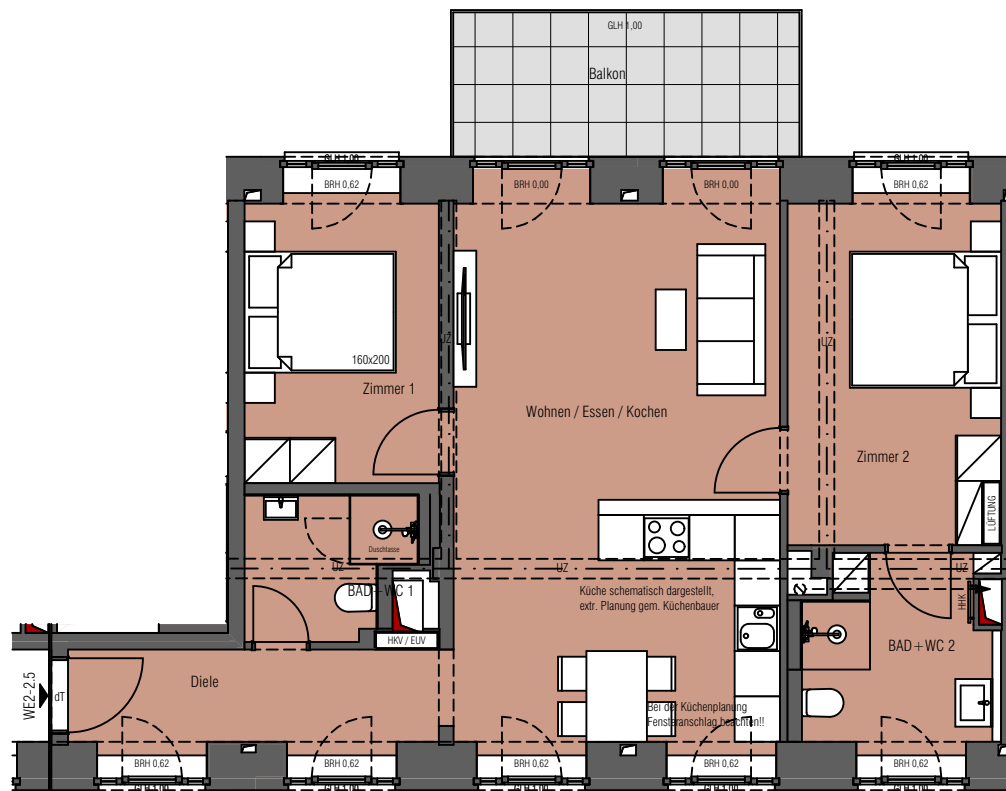
2.Obergeschoss
