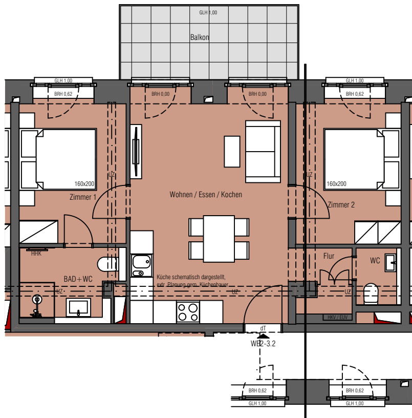
3.Obergeschoss
