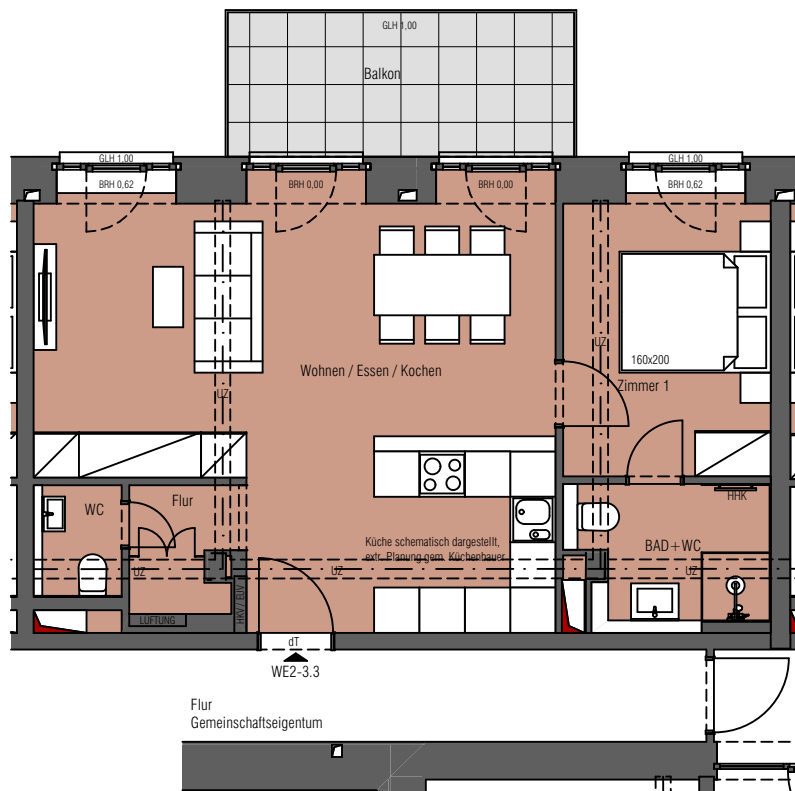
3.Obergeschoss
