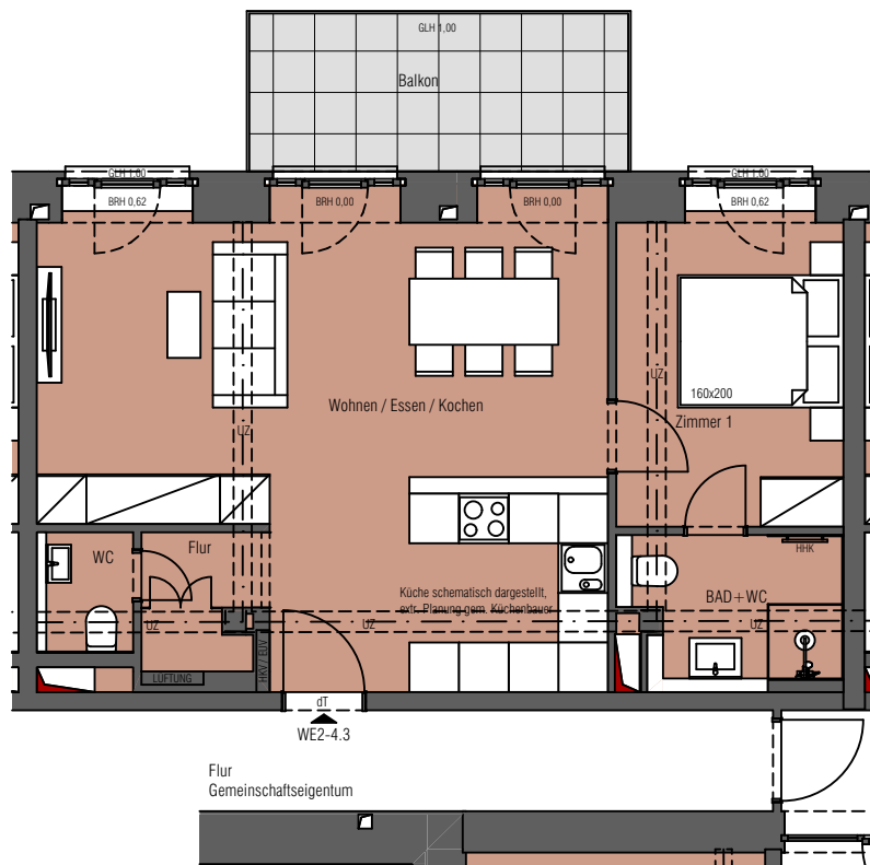
4.Obergeschoss
