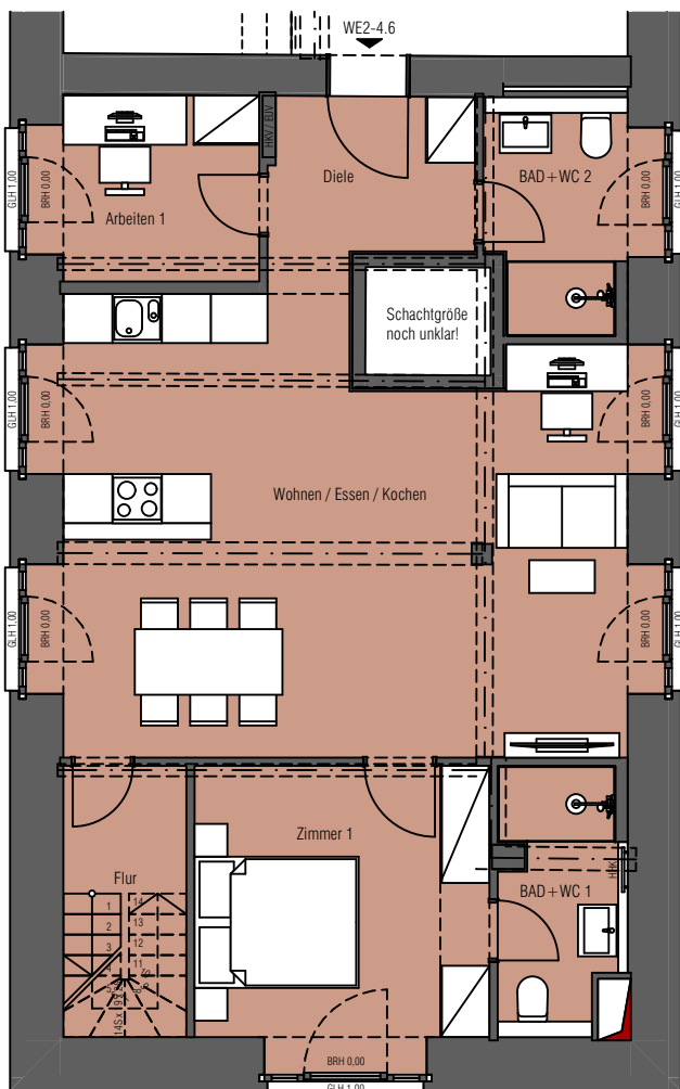
4.Obergeschoss
