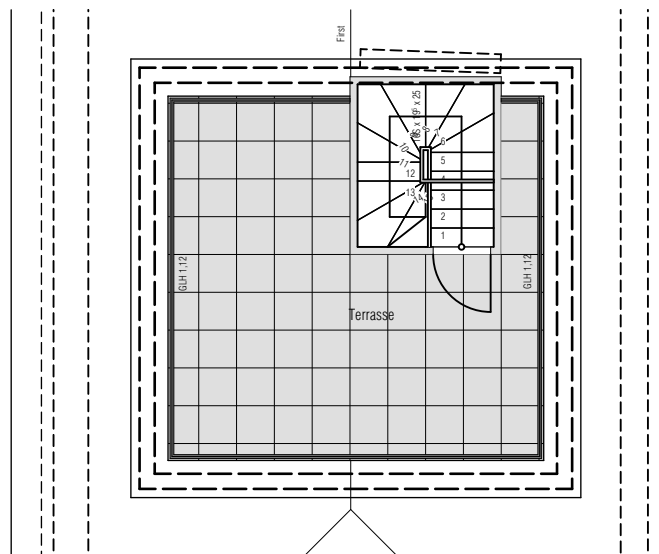
Dachaufsicht
