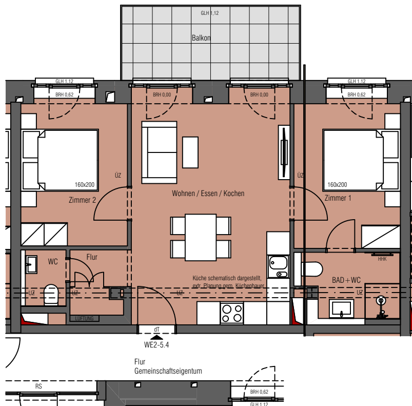
5.Obergeschoss
