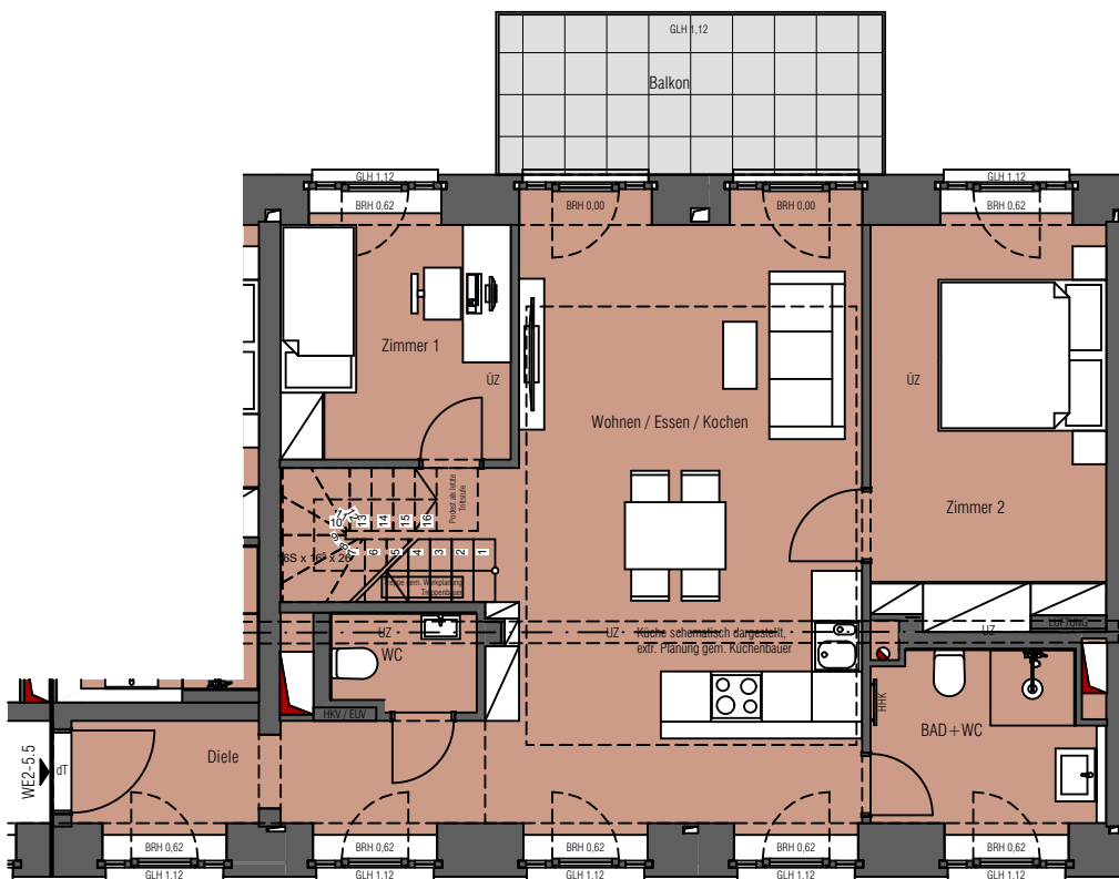
5.Obergeschoss
