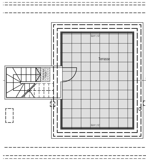
Dachaufsicht
