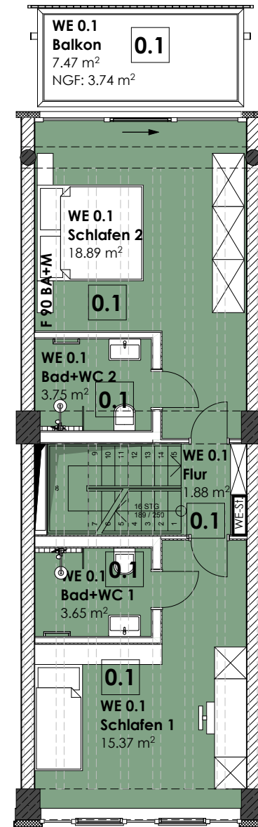
1. Obergeschoss
