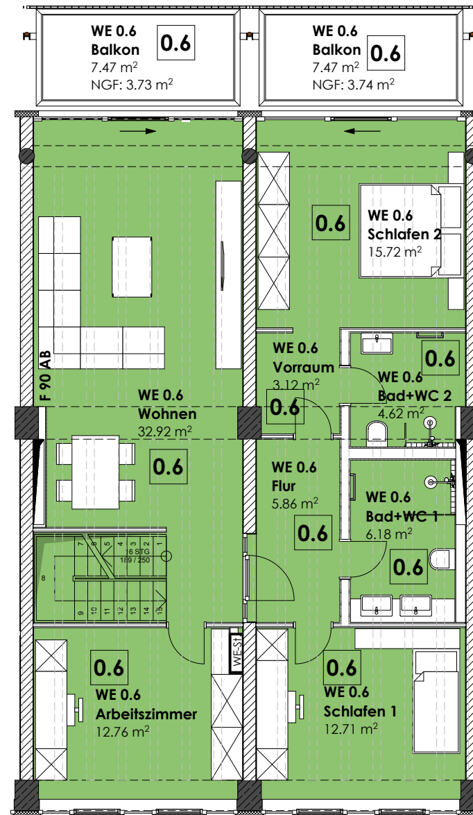
1. Obergeschoss
